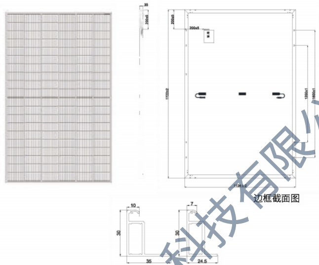
尺寸图纸 (mm)
